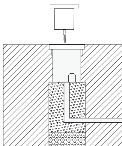
Схема монтажа
